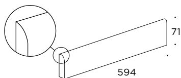
Battiscopa 60 ≠12 mm
